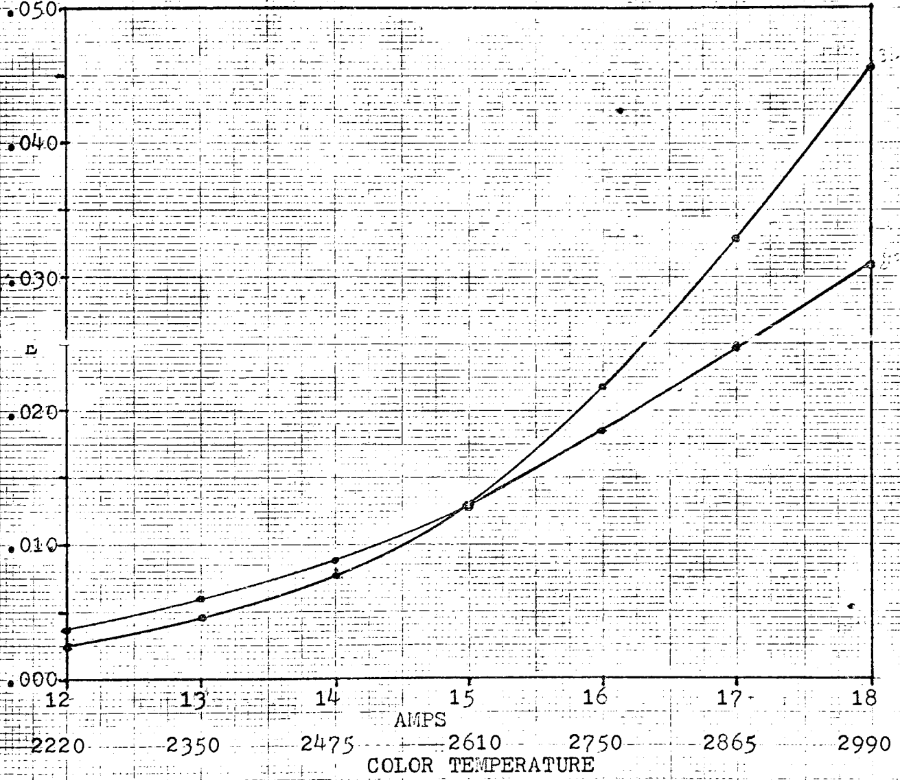
FIG. 15. E vs AMPS
